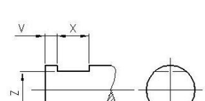
Type 11: 1-nøgleflade
