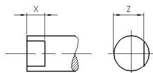
Type 8: 1-nøgleflade
