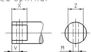
Type 11: 1-nøgleflade
