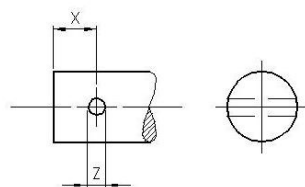
Type 8: 1-nøgleflade
