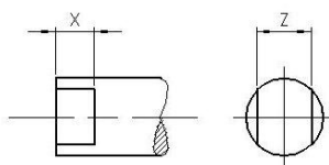
Type 1: 2-nøgleflader
