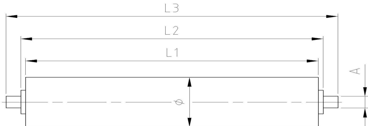
Type 1: 2-nøgleflader
