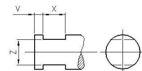
Type 9: 2-nøgleflader
