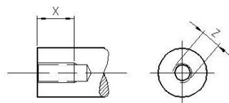
Type 2: indv. gevind
